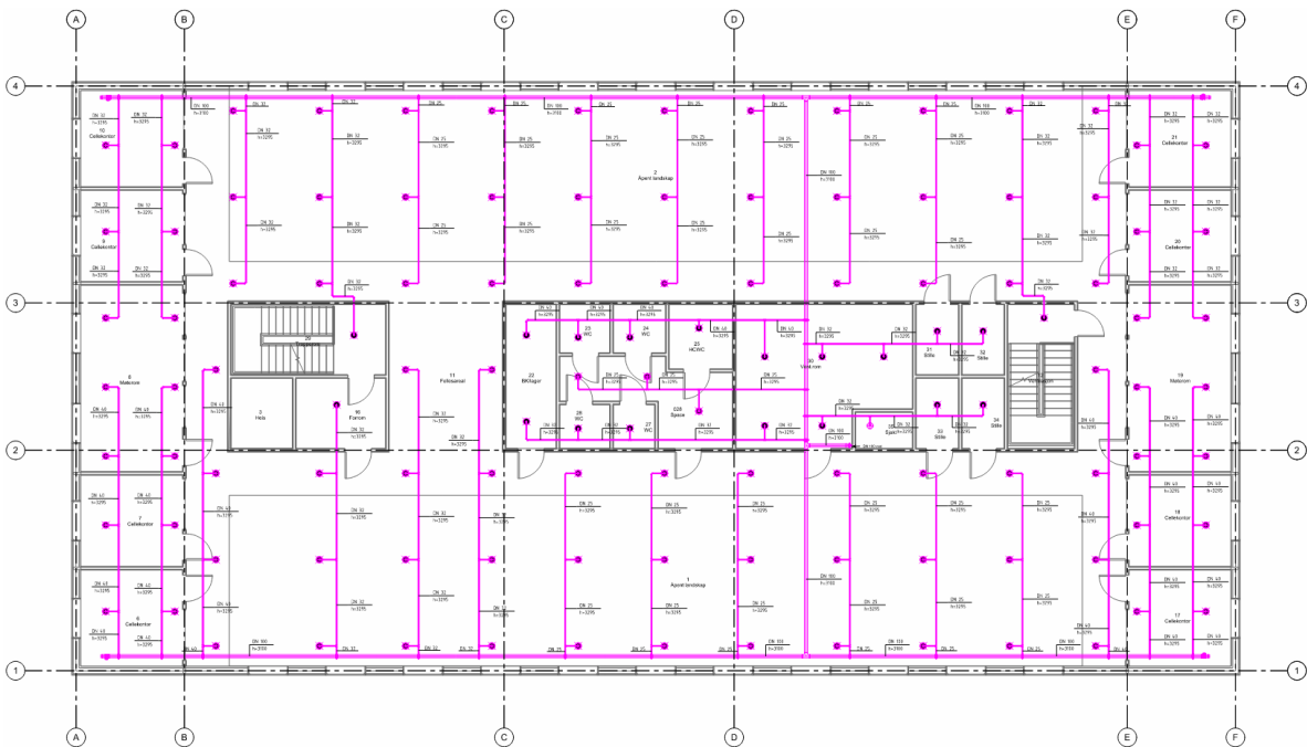
Figur 2 - Plantegning av et konvensjonelt sprinkleranlegg for kontor hvor anlegget er fargelagt rosa, med dyser som sirkler og rørstrekk som linjer.
