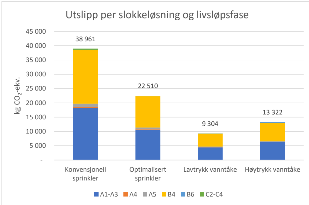
Figur 9 - Totale klimagassutslipp for hvert alternativ og livsløpsfase. Livsløpsfaser: A1-A3 Produktstadiet, A4-A5 Transport og byggeglass, B4 Utskifting, B6 Energibruk i drift og C2-C4 Livsløpets sluttstadium.
