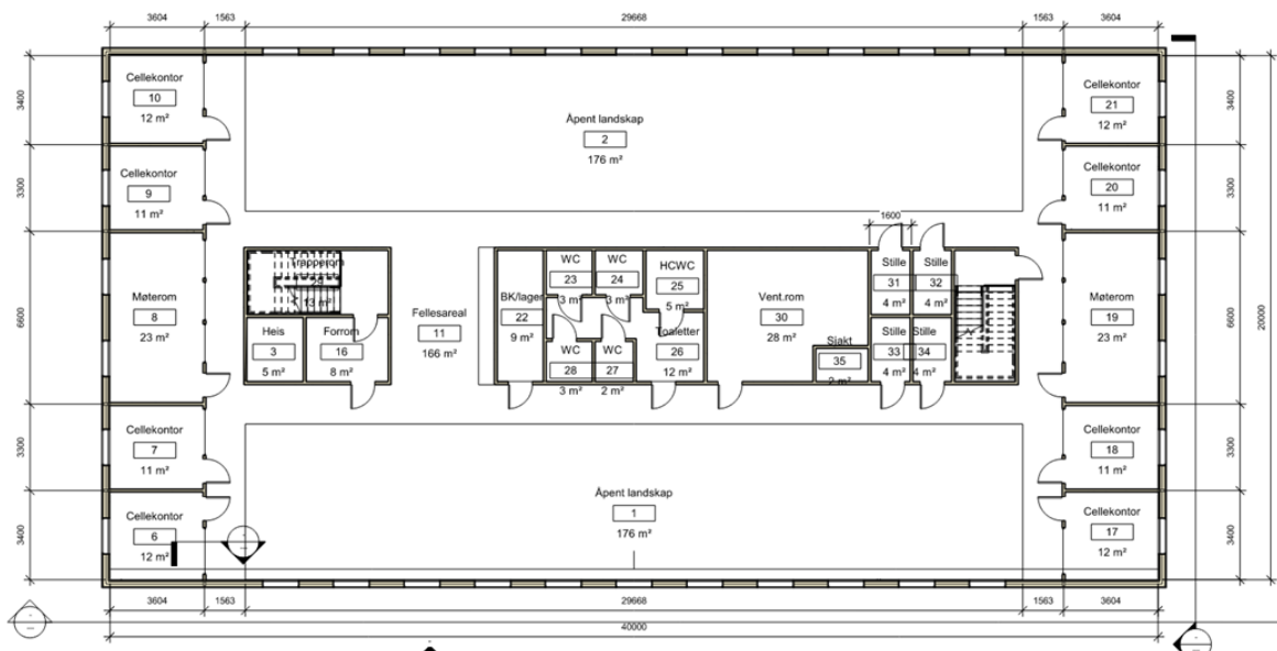
Figur 1 - Den generiske kontoretasjen som brukes som underlag ved sammenligning av brannsløkkeløsninger.
